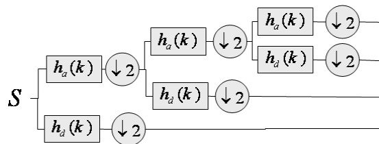
شکل ۲- درخت موجک گسسته دوتائی با ۴ زیرباند نامساوی
