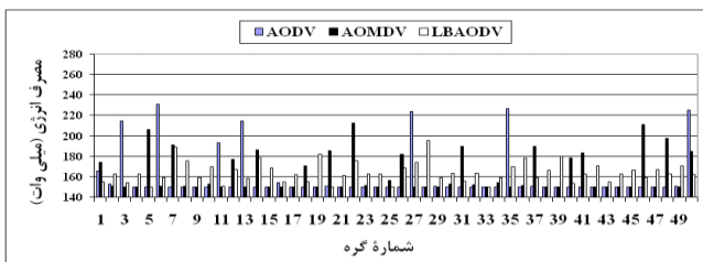
شکل (۱۰): مصرف انرژی گره ها (حداکثر سرعت: 15 Km/h)
