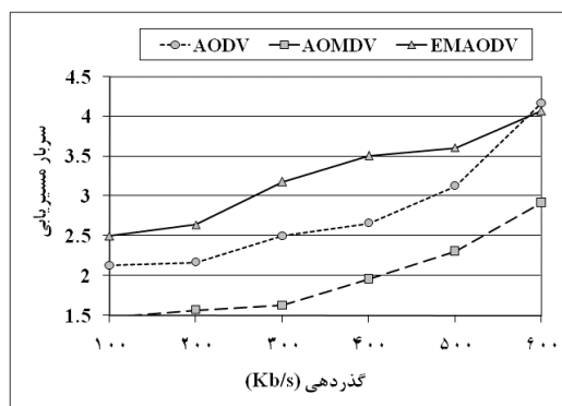
شکل (۷): سر بار مسیریابی در برابر نرخ ارسال
