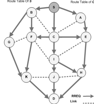
شکل (۱): فرآیند انتشار بسته درخواست مسیر
