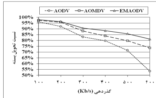
شکل (۵): نسبت تحویل بسته در برابر گذردهی
